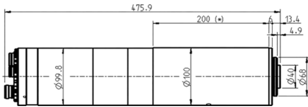
Abmessungen
